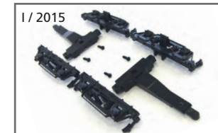
36052 Drehgestell für US Personenwagen, 1 Paar American Passenger Trucks, 1 pair
